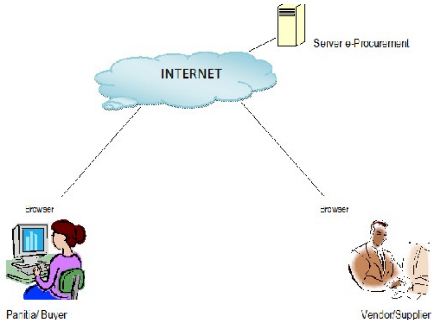
Gambar. 1 Arsitektur Procuriza
